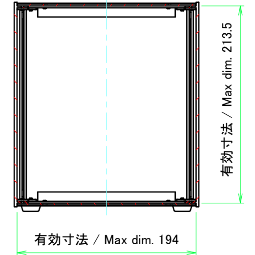
C-C ( 1 : 4 )
