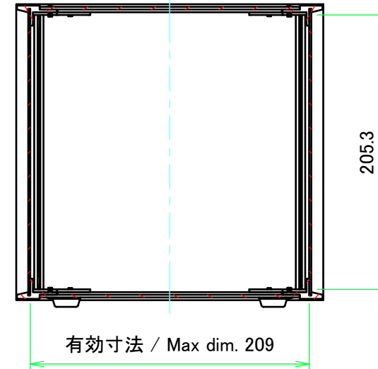
A-A ( 1 : 4 )
