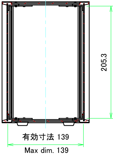
A-A (1:4)
