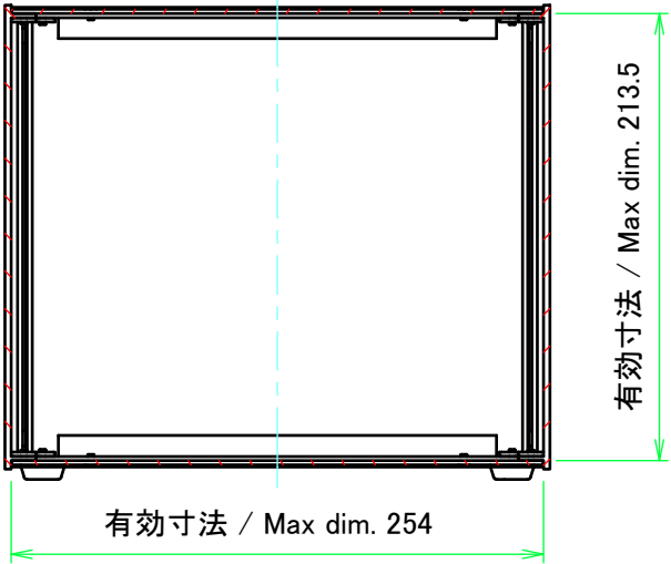
C-C ( 1 : 4 )
