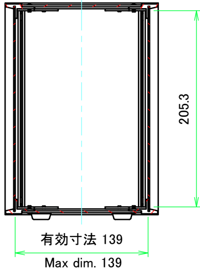
A-A ( 1 : 4 )
