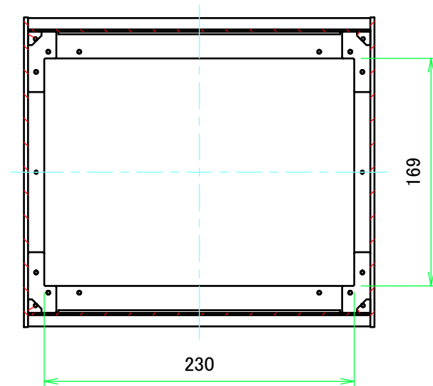
B-B ( 1 : 4 )
