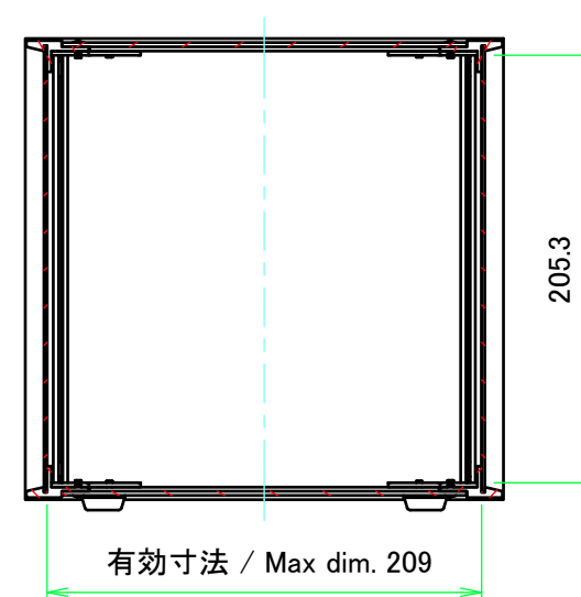
A-A ( 1 : 4 )
