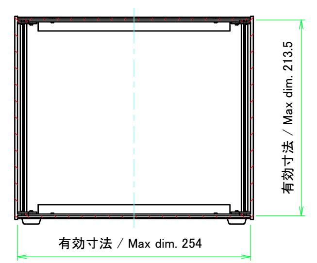
C-C ( 1 : 4 )
