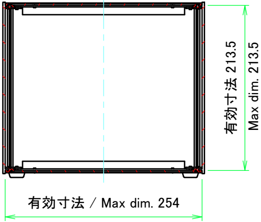
C-C ( 1 : 5 )
