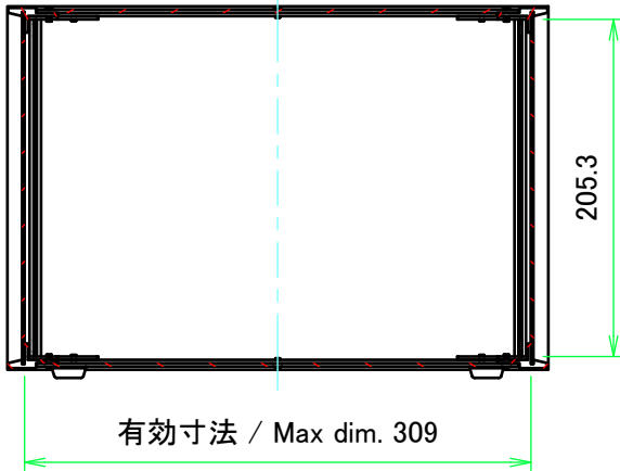
A-A ( 1 : 5 )
