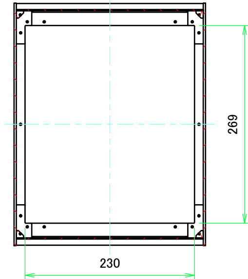
B-B ( 1 : 5 )
