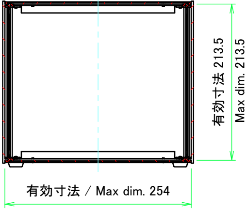
C-C ( 1 : 5 )
