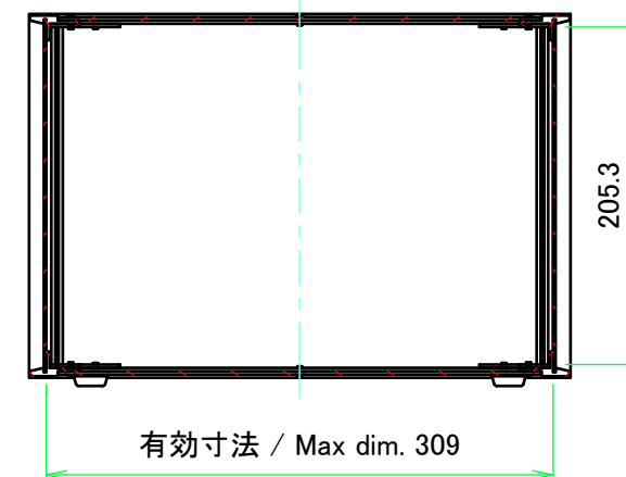
A-A (1:5)
