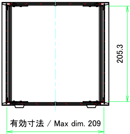
A-A (1:5)
