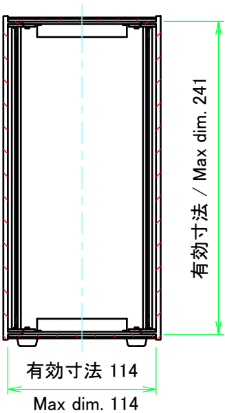
C-C ( 1 : 4 )
