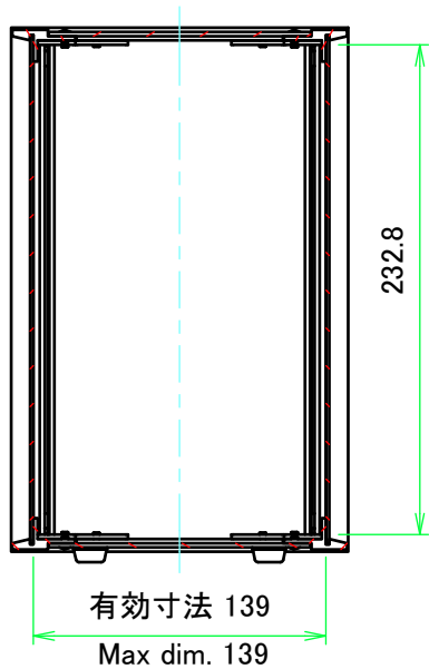
A-A ( 1 : 4 )
