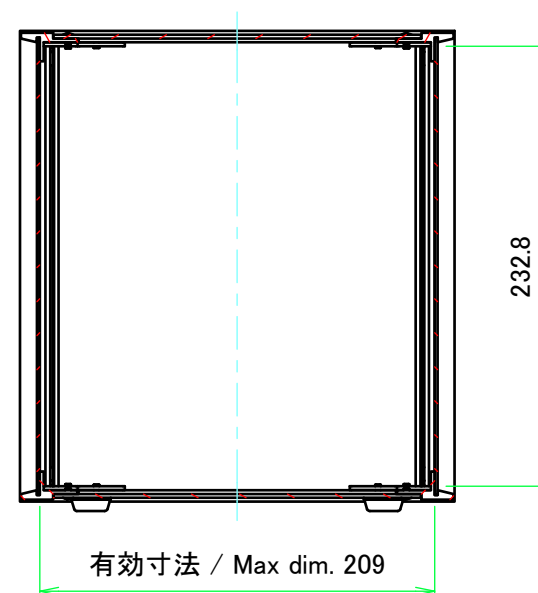
A-A ( 1 : 4 )
