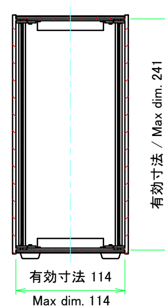
C-C ( 1 : 4 )
