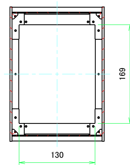
B-B ( 1 : 4 )
