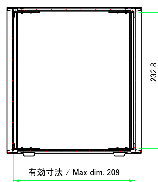
A-A ( 1 : 4 )
