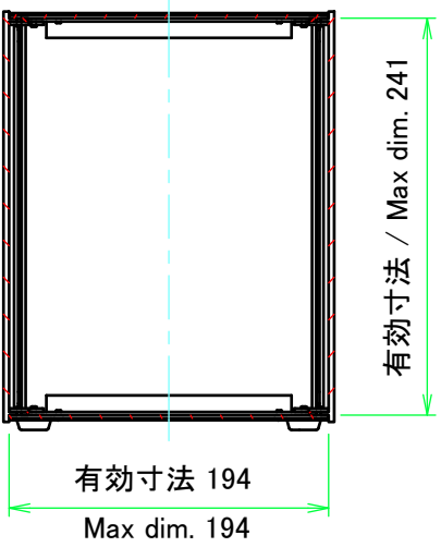
C-C ( 1 : 5 )
