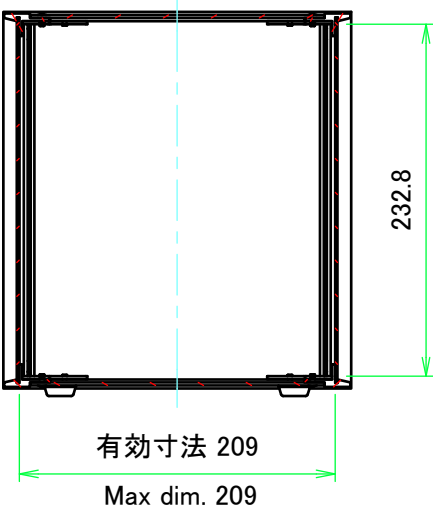
A-A ( 1 : 5 )
