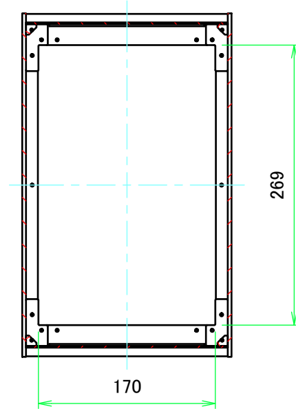
B-B ( 1 : 5 )
