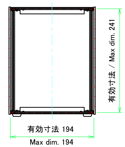
C-C ( 1 : 5 )
