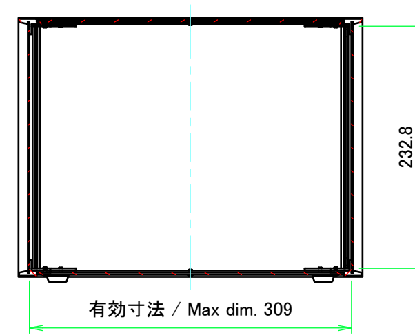
A-A ( 1 : 5 )
