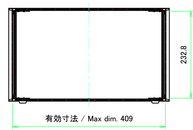
A-A (1:6)
