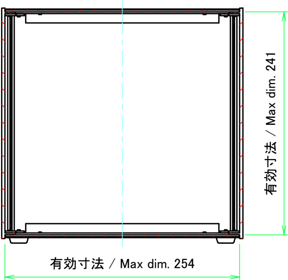
C-C ( 1 : 4 )
