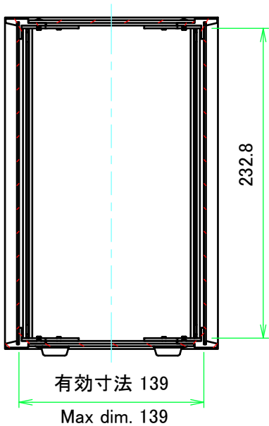
A-A ( 1 : 4 )
