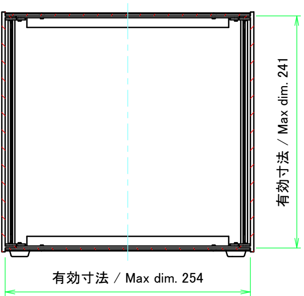
C-C ( 1 : 4 )
