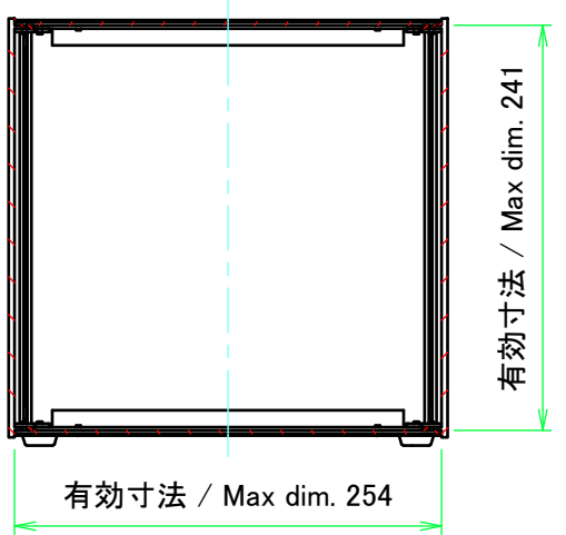
C-C ( 1 : 5 )
