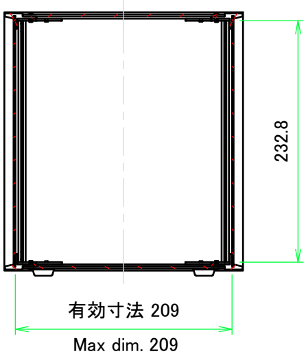
A-A ( 1 : 5 )
