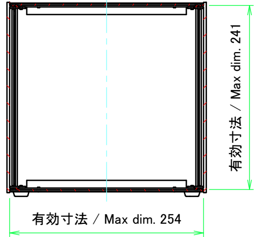
C-C ( 1 : 5 )
