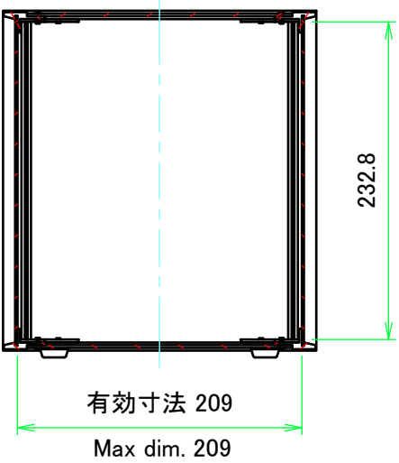
A-A ( 1 : 5 )
