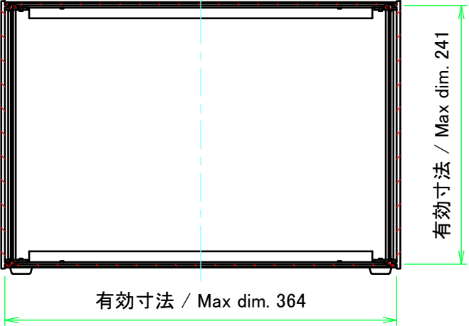
C-C ( 1 : 5 )
