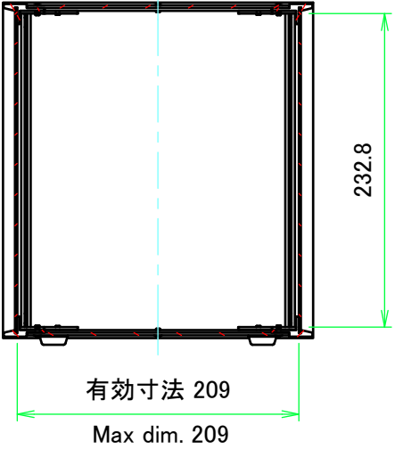
A-A (1:5)
