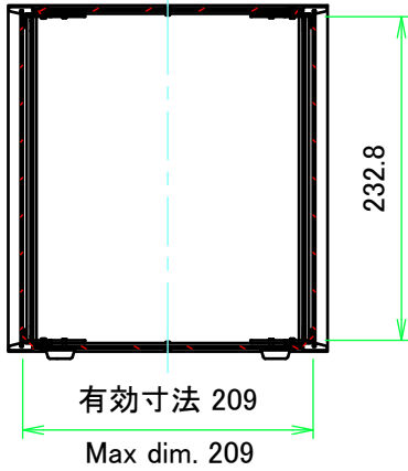
A-A (1:6)
