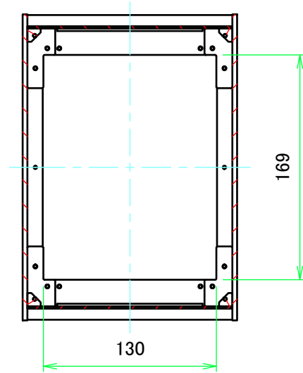
B-B ( 1 : 4 )
