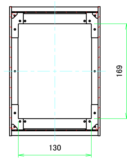
B-B ( 1 : 4 )
