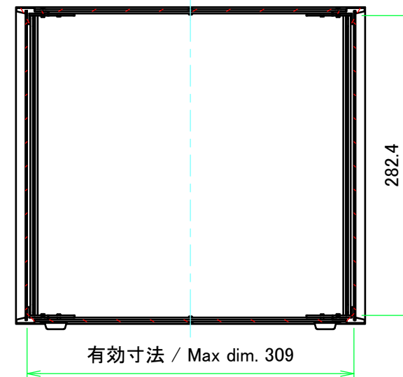
A-A ( 1 : 5 )
