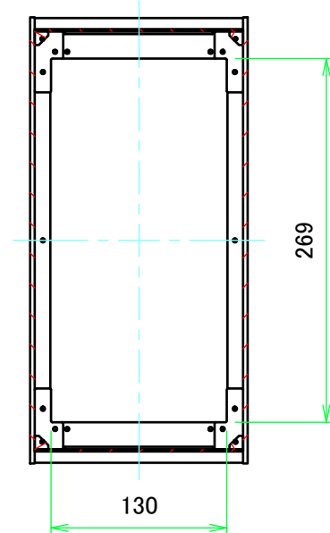
B-B ( 1 : 5 )
