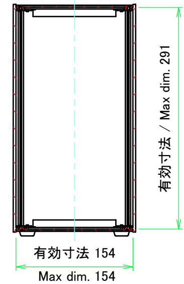
C-C ( 1 : 5 )
