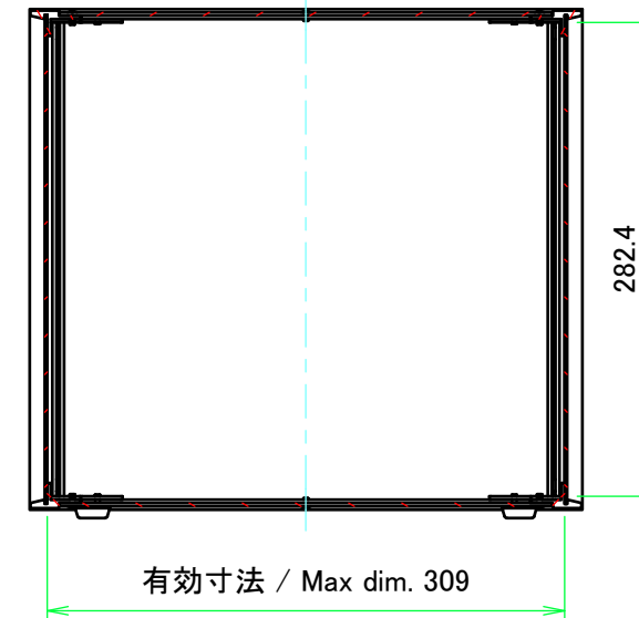
A-A ( 1 : 5 )
