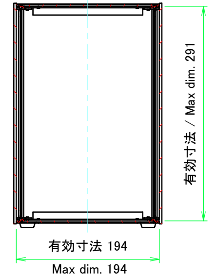
C-C ( 1 : 5 )
