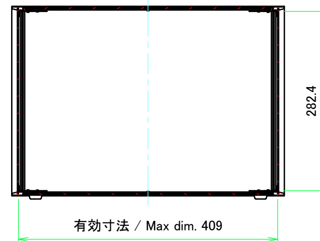
A-A (1:6)
