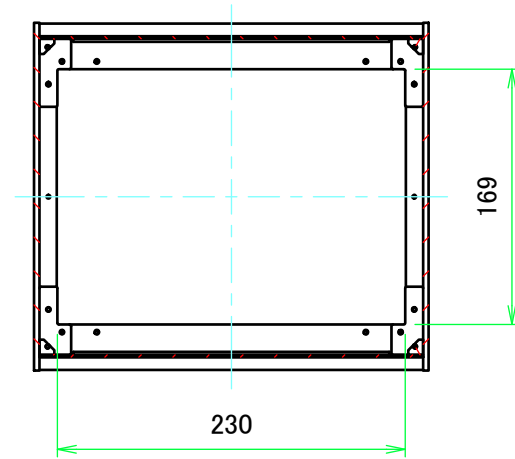
B-B ( 1 : 5 )
