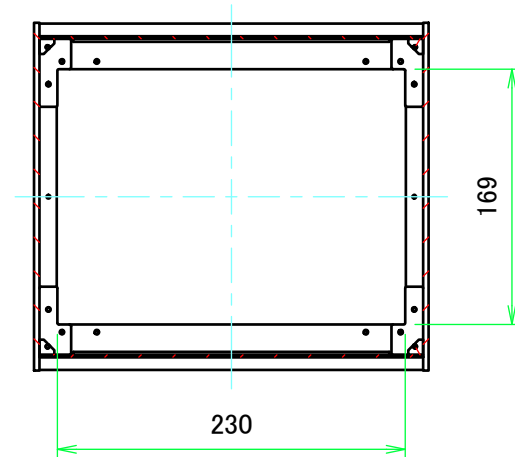
B-B ( 1 : 5 )
