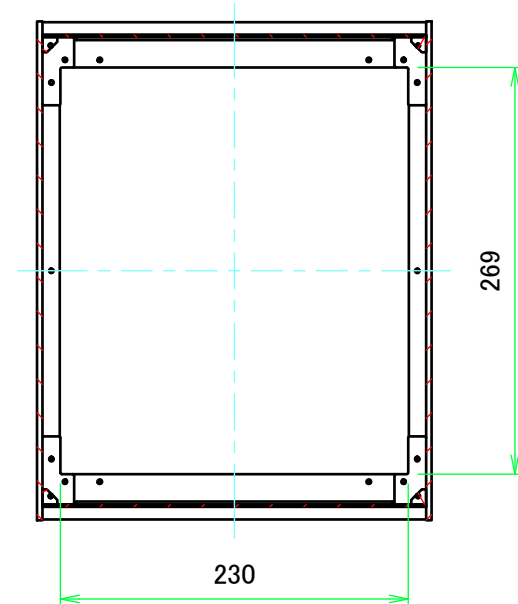
B-B ( 1 : 5 )
