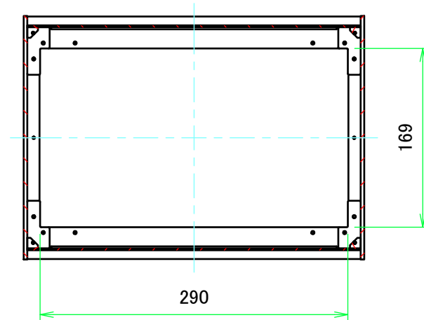
B-B ( 1 : 5 )
