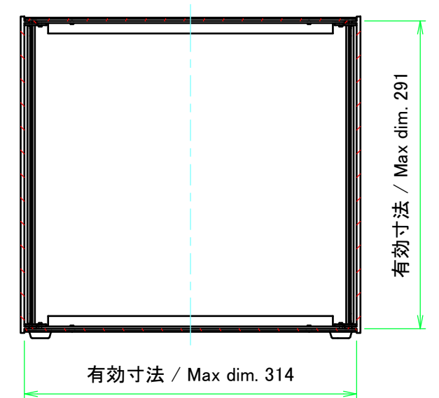
C-C ( 1 : 5 )
