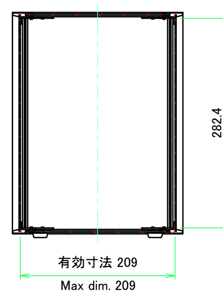
A-A ( 1 : 5 )
