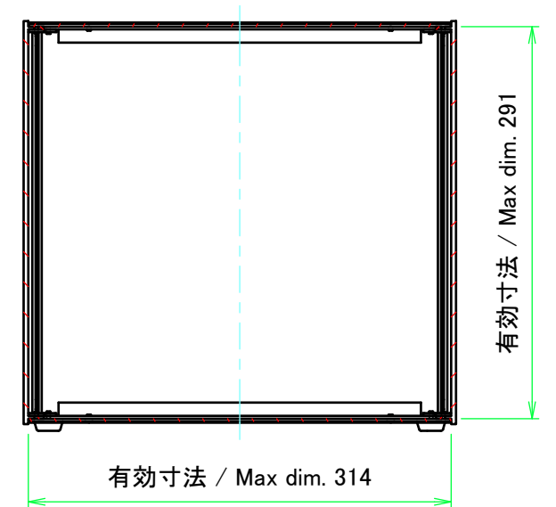
C-C ( 1 : 5 )
