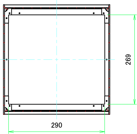
B-B ( 1 : 6 )
