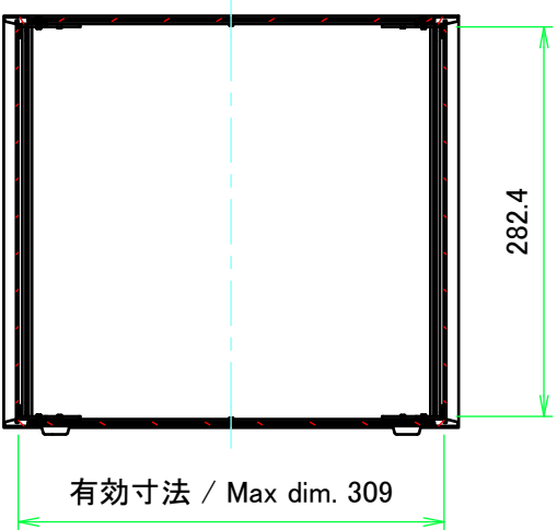
A-A ( 1 : 6 )
