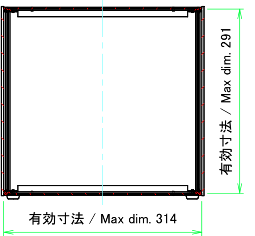
C-C ( 1 : 6 )
