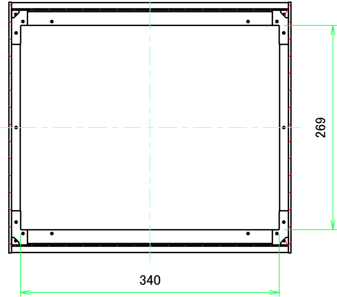
B-B ( 1 : 5 )
