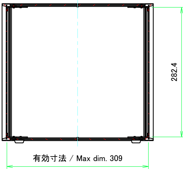
A-A ( 1 : 5 )
