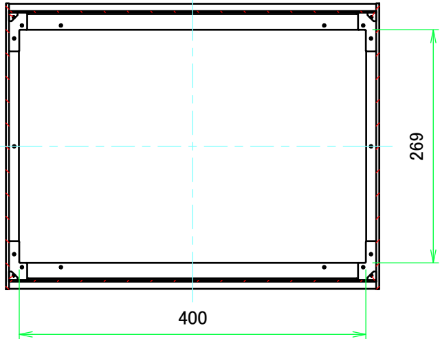
B-B ( 1 : 6 )
