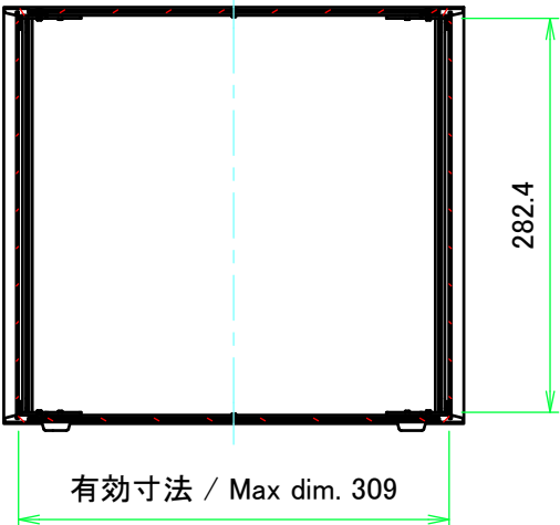
A-A ( 1 : 6 )
