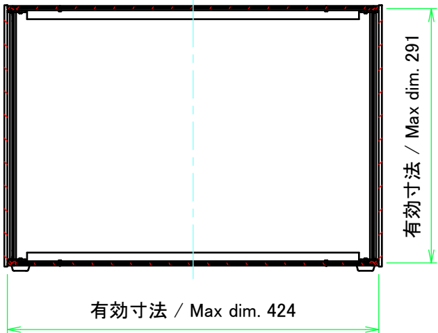
C-C ( 1 : 6 )
