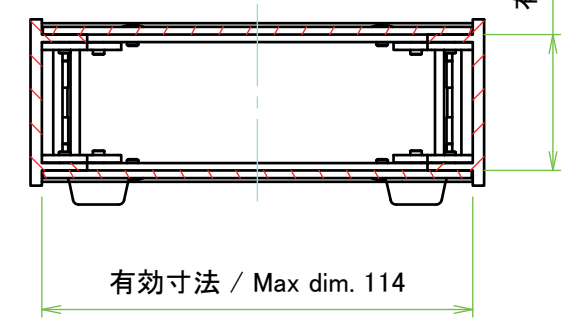
C-C (1:2)
