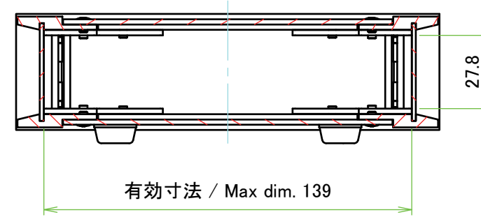
A-A (1:2)
