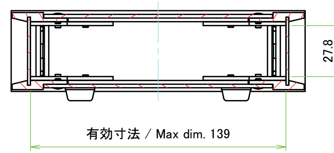
A-A ( 1 : 2 )
