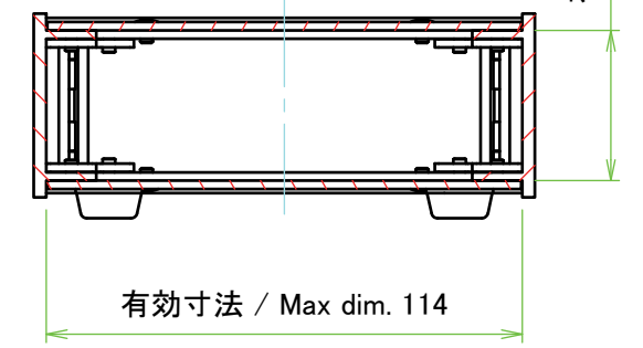
C-C ( 1 : 2 )
