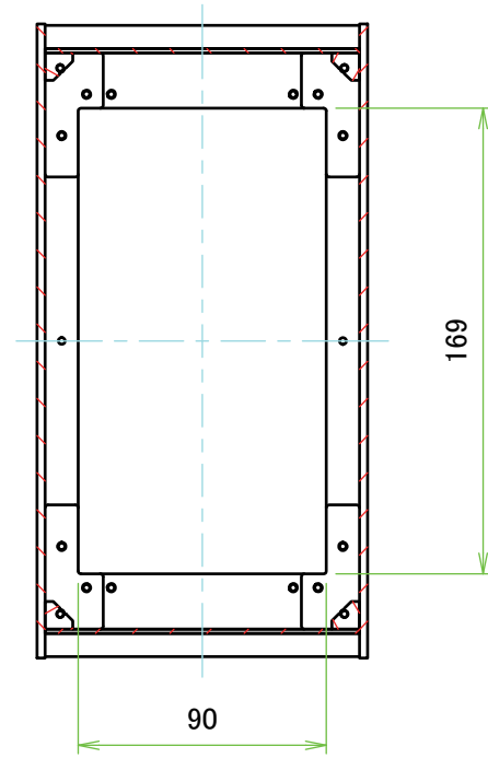
B-B ( 1 : 3 )
