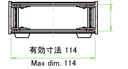
C-C ( 1 : 3 )
