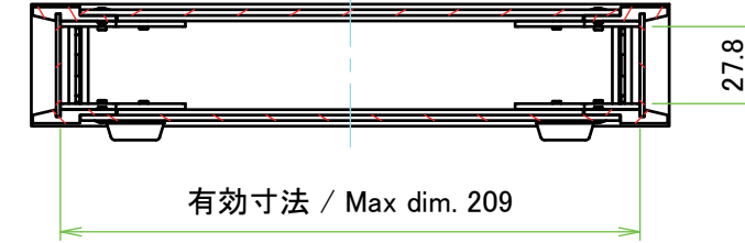
A-A ( 1 : 3 )
