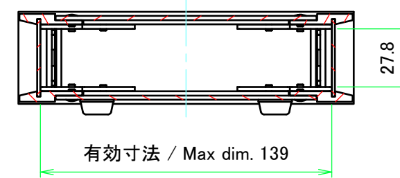
A-A ( 1 : 2.5 )
