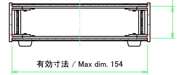
C-C ( 1 : 2.5 )
