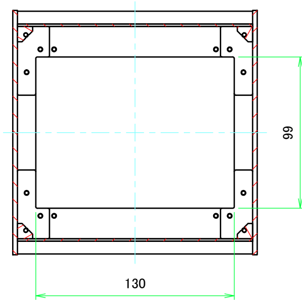
B-B ( 1 : 2.5 )
