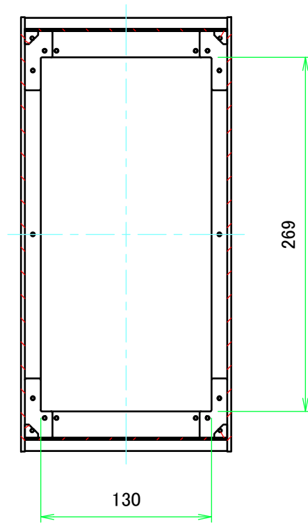
B-B ( 1 : 4 )
