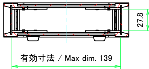
A-A (1:3)
