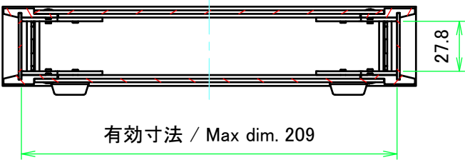
A-A ( 1 : 3 )
