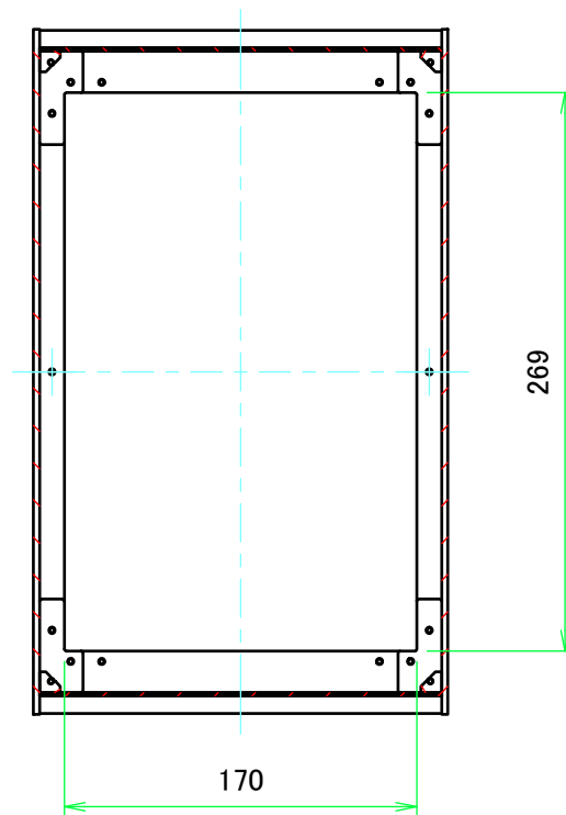
B-B ( 1 : 4 )
