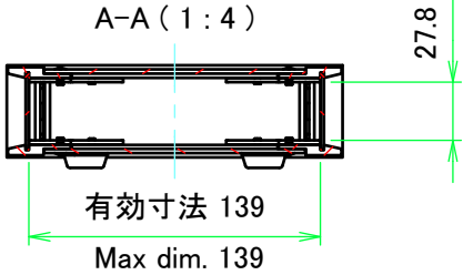
A-A ( 1 : 4 )
