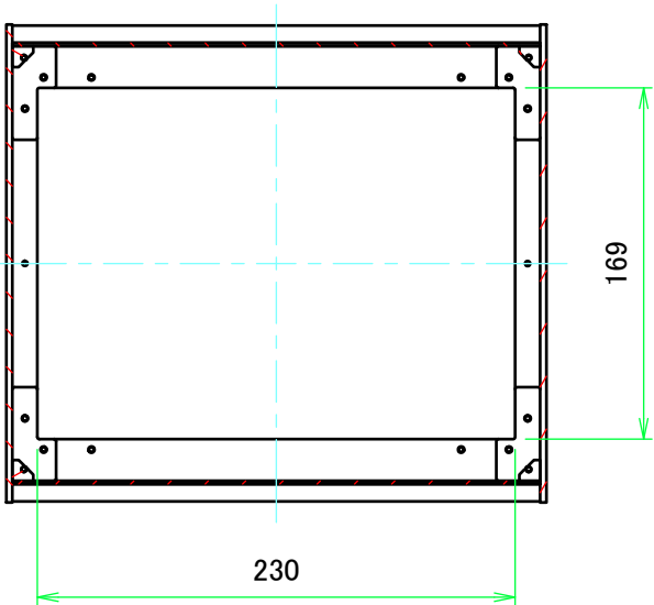
B-B ( 1 : 4 )
