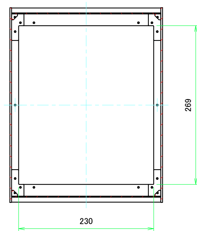
B-B ( 1 : 4 )
