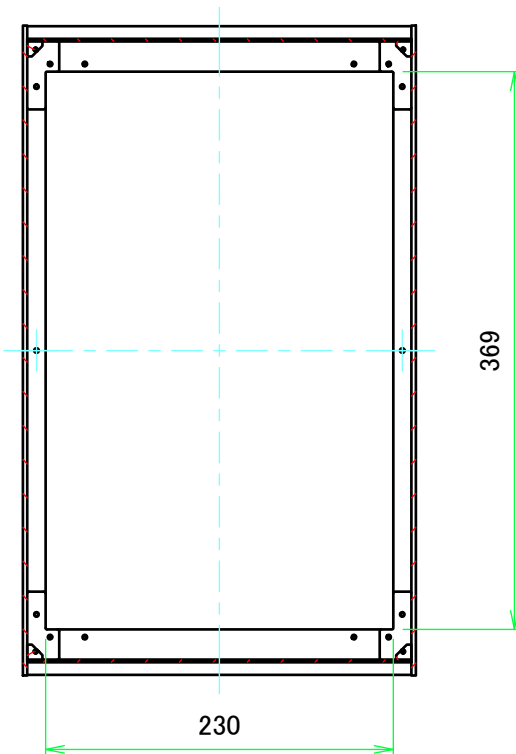
B-B ( 1 : 5 )
