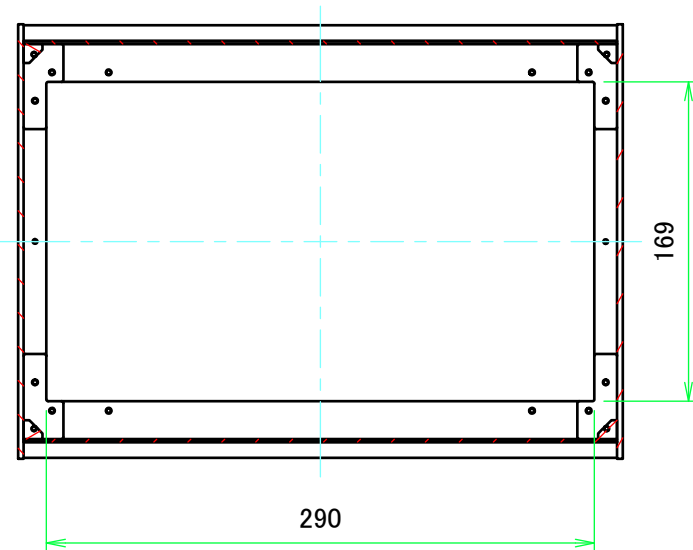
B-B ( 1 : 4 )
