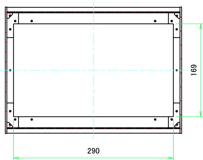
B-B ( 1 : 4 )
